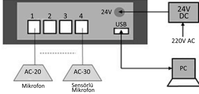
Bağlantı Şeması:
